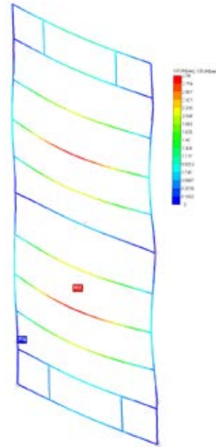
Диаграмма прогибов
